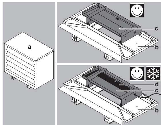
a Capac pentru reducerea zgomotului b Componentele din partea de jos a capacului pentru reducerea nivelului sunetului c Set tavă de evacuare d Încălzitor tavă de evacuare
