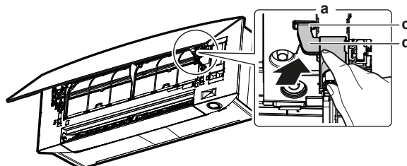
a Fața posterioară a panoului frontal
