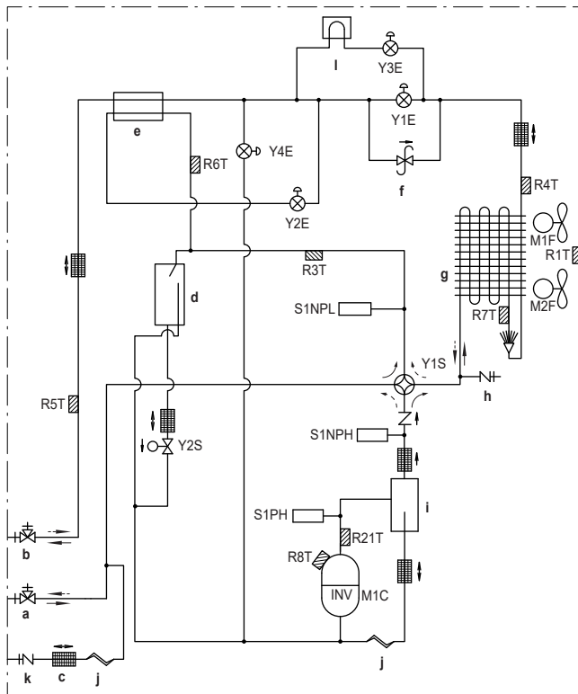
Schema tubaturii: 10+12 HP
