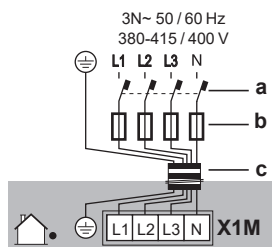
a Întreruptor pentru scurgeri la pământ b Siguranță c Cablu de alimentare de la rețea
