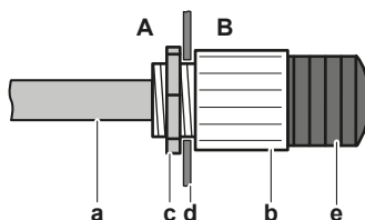
A Interiorul unității exterioare B Exteriorul unității exterioare a Cablu b Bucșă c Piuliță d Cadru e Tub
