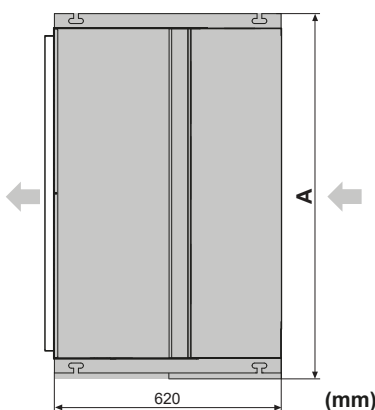
12-1 Dimensiunea deschiderii tavanului (A)
