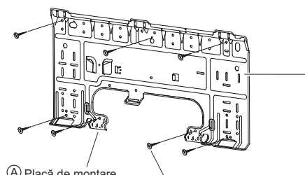
Ⓐ Placă de montare
