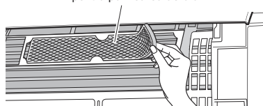
Ⓑ Filtru fotocatalitic din apatit de titan pentru purificarea aerului (2)
