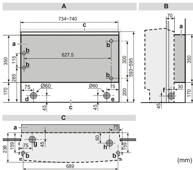
5-3 Desenul de instalare de instalare a unității interioare: Instalație semimască
