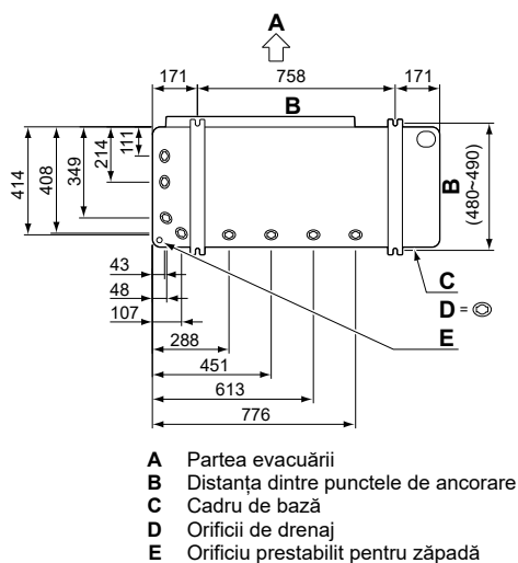
Orificii de drenaj (dimensiuni în mm)
