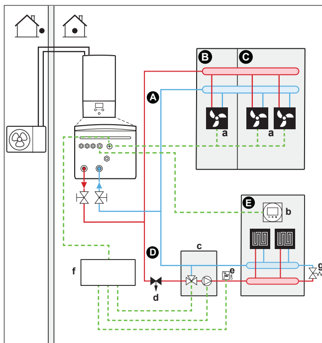
2 Sistem cu separator hidraulic pentru zona principală:
