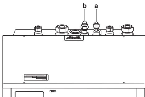
a Racordul agentului frigorific lichid b Racordul agentului frigorific gazos
