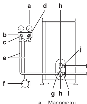
a Manometru
