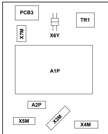
Poziția în cutia de distribuție a compresorului
