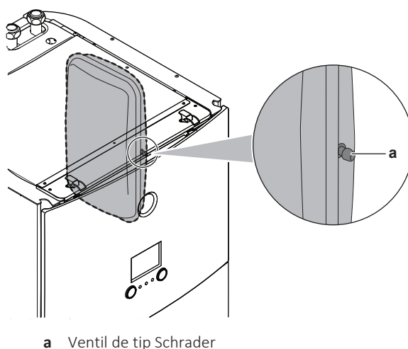
a Ventil de tip Schrader
