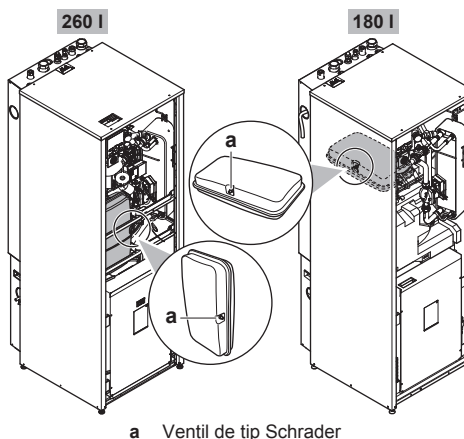
a Ventil de tip Schrader
