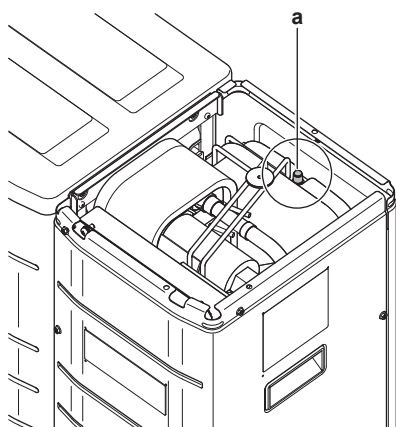
a Ventil de tip Schrader
