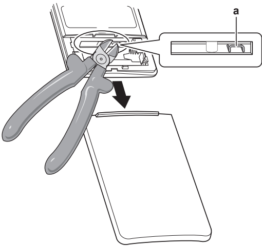
a Șuntul de adresă J4
